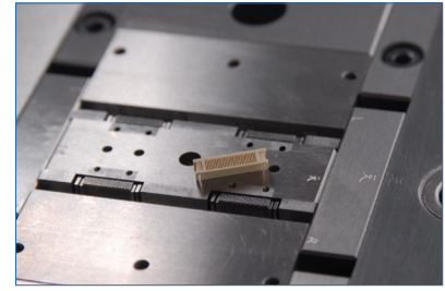
Khuôn nhựa có độ chính xác cao
